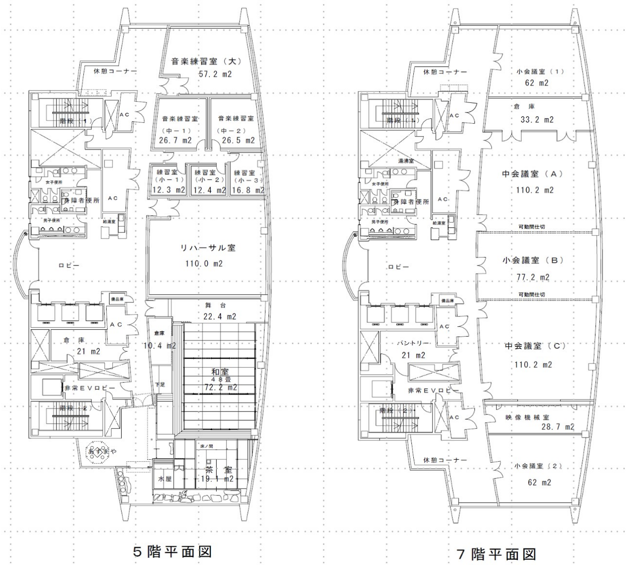
【図4-2】 清水テルサ5階・7階平面図
