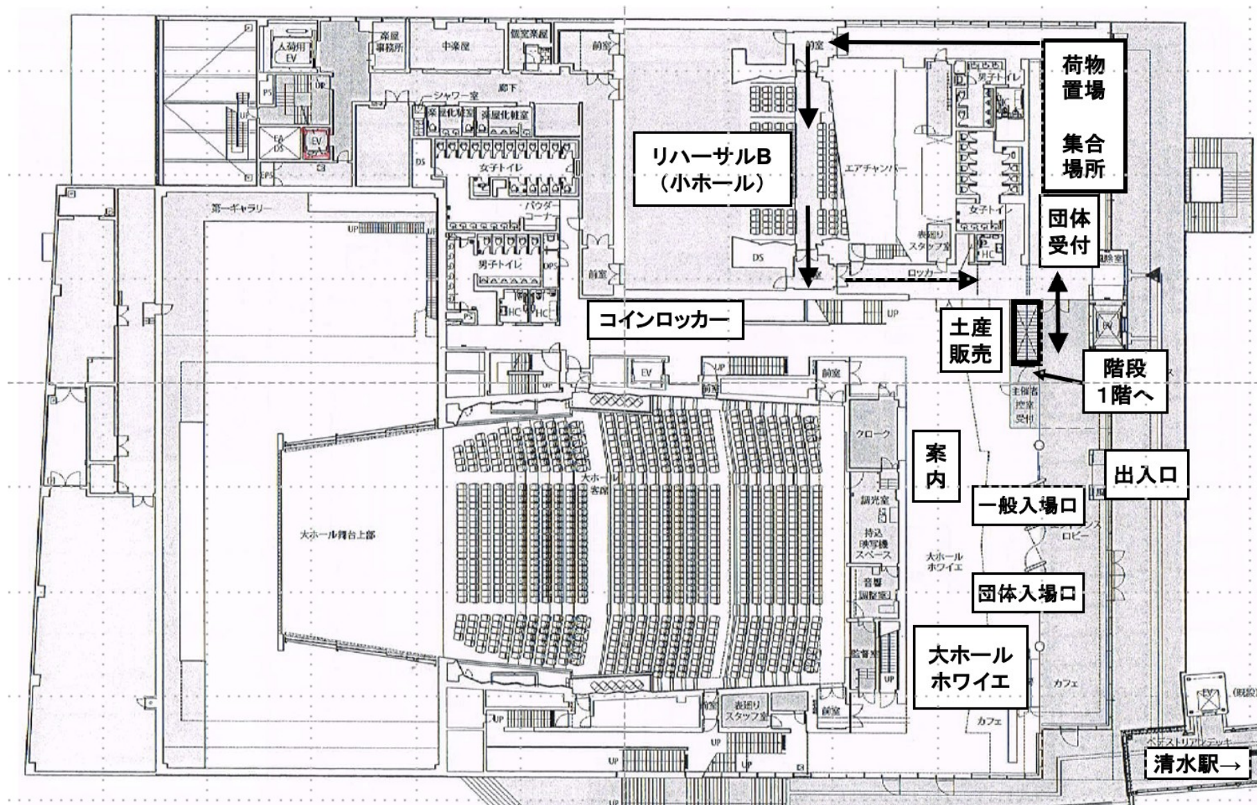
【図2-2】清水マリナート2階平面図
